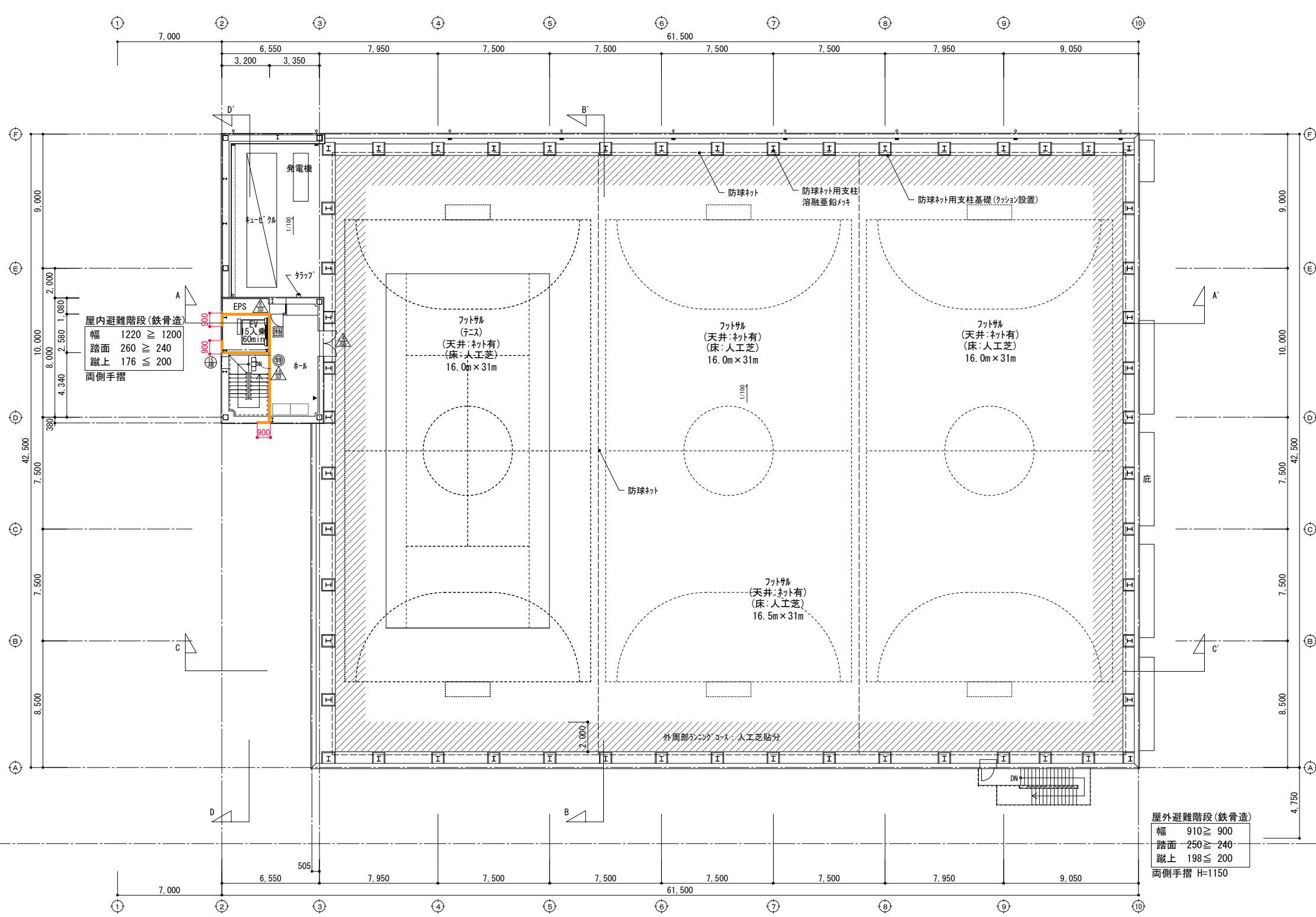
R階平面図 A1:S=1/150 A3:S=1/300
